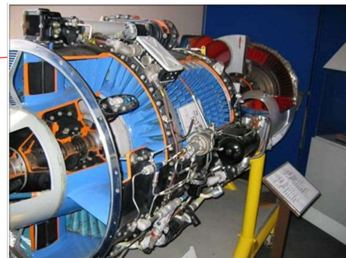
Orenda 11
